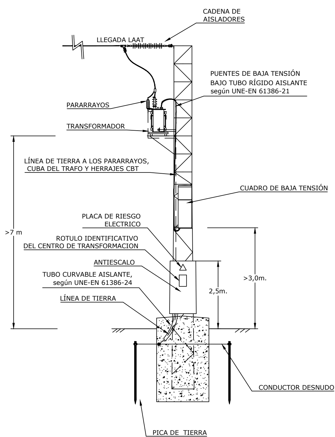
VISTA LATERAL
