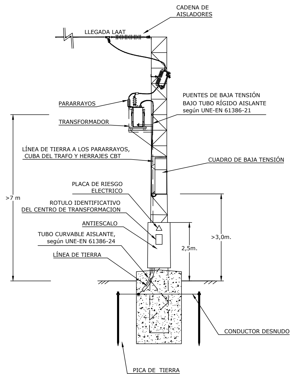
VISTA LATERAL
