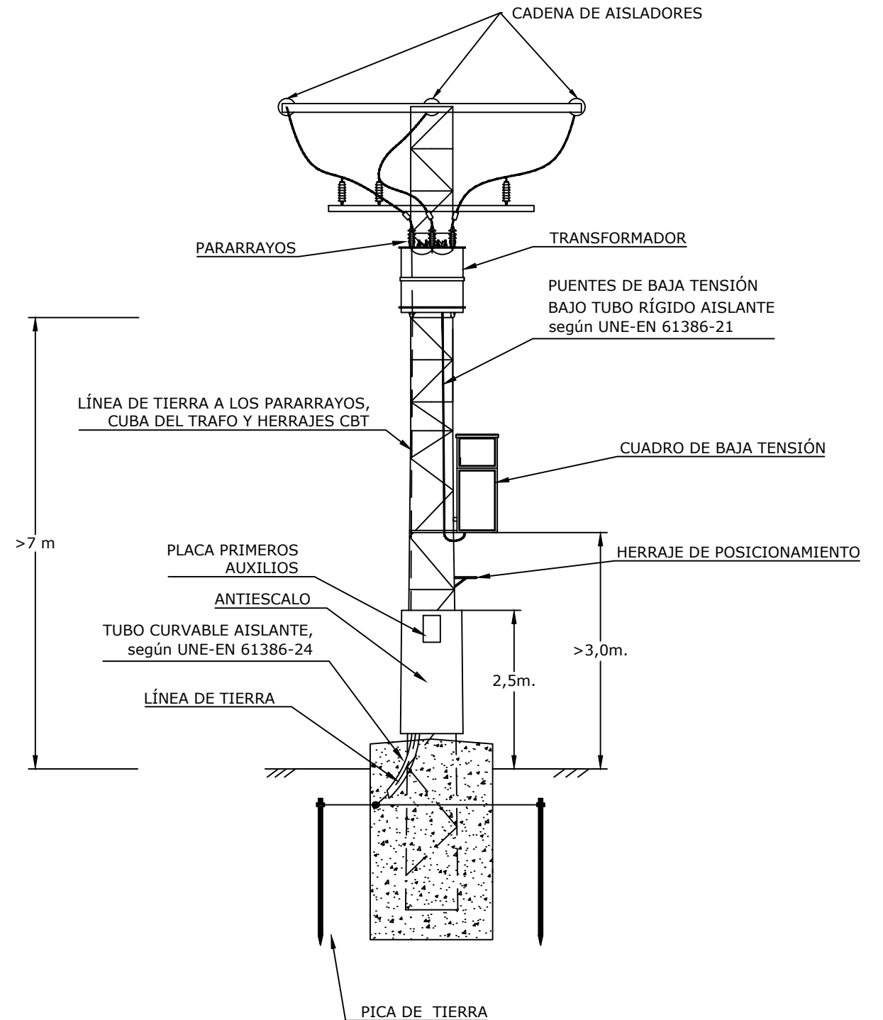
ALZADO
