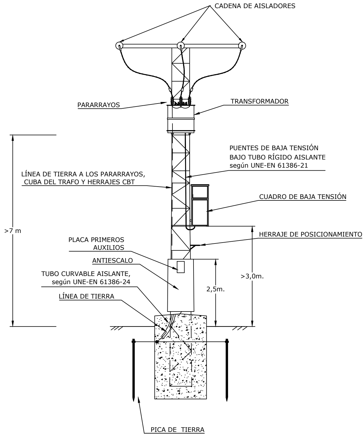
ALZADO
