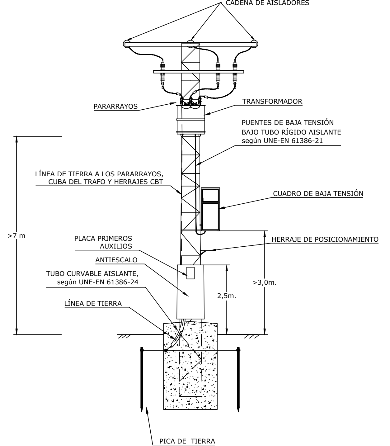
ALZADO
