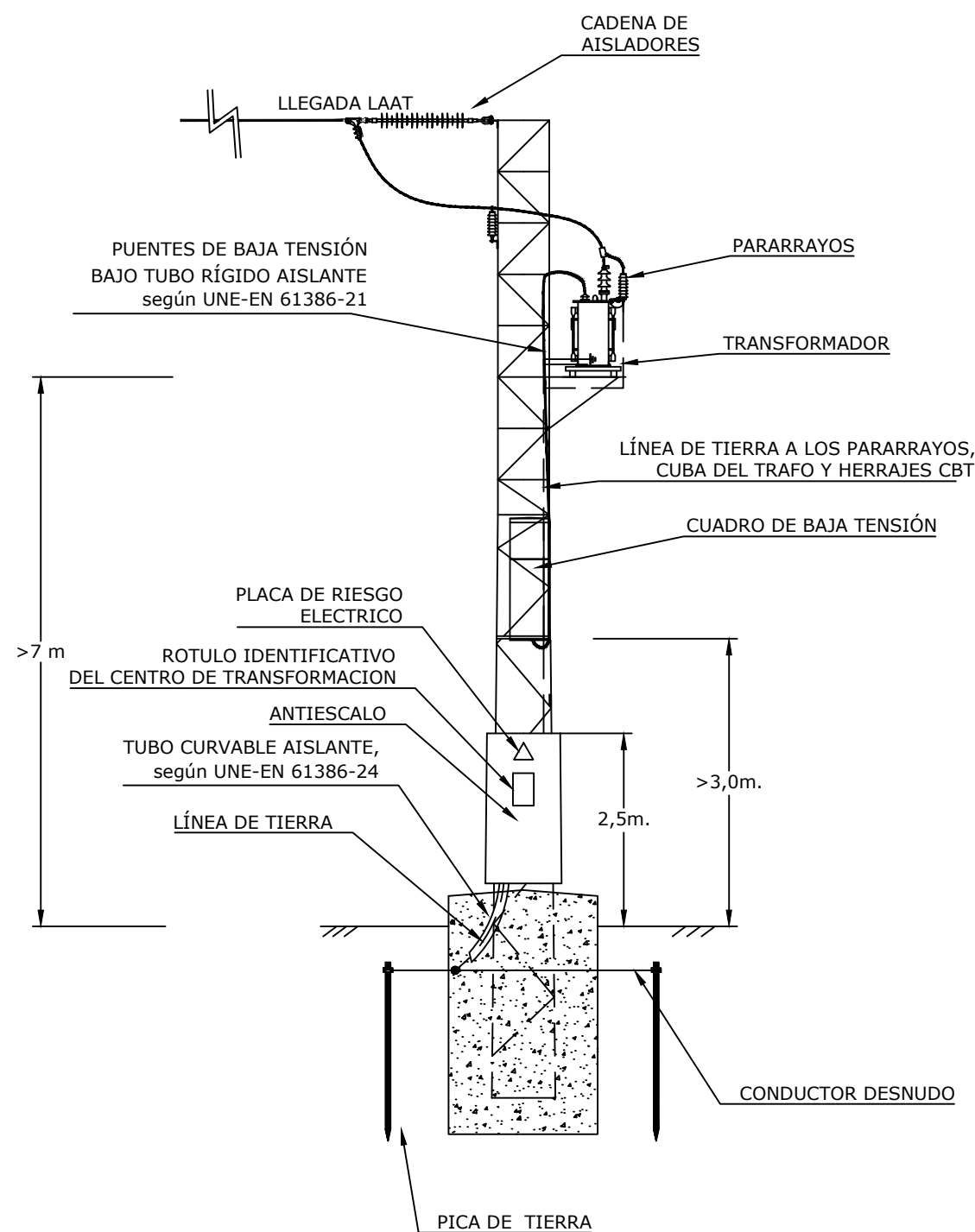
VISTA LATERAL
