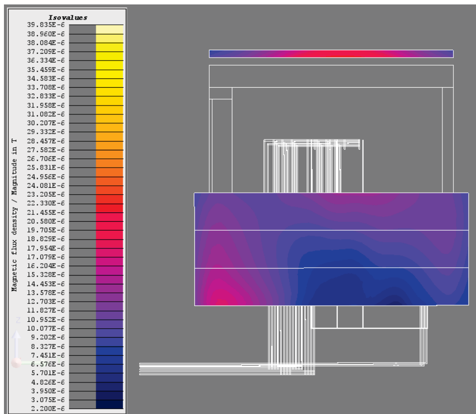
Figura 23. Densidad de flujo magnético ( B[T] = \text{Magnitud } B ) en el panel derecho (2L+2T).
