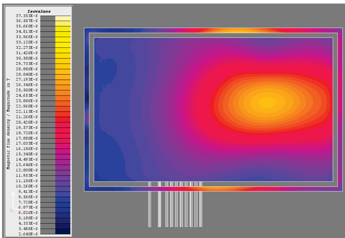
Figura 10. Densidad de flujo magnético ( B[T] = \text{Magnitud } B ) en el panel techo (2L+1T).
