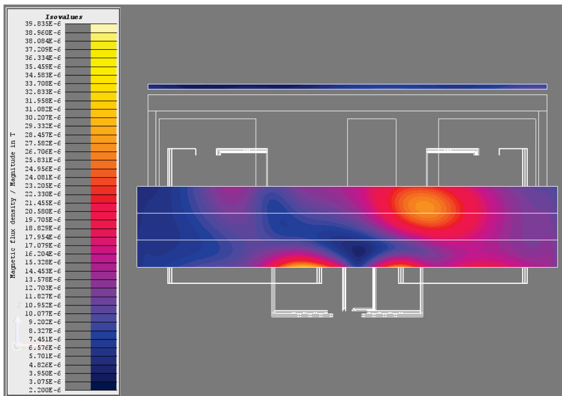
Figura 22. Densidad de flujo magnético ( B[T] = \text{Magnitud } B ) en el panel frontal (2L+2T).
